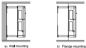
Abbildung 3-2 Installation
