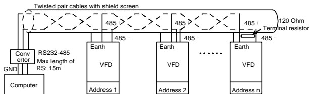
Abbildung 7.2 Praktisches Anwendungsschema der Chrysanthemenschaltung
