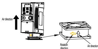
Abbildung 6-1 Lüftereinbau bei Frequenzumrichtern 1PH, 230 V, ≤2,2 kW
