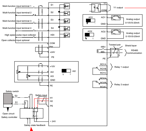
Abbildung 3-10 Verdrahtung des Steuerkreises für Frequenzumrichter \geq 1,5 kW (3PH 230 V) & \geq 4 kW (3PH 400 V)
