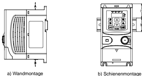
Abbildung 3-1 Installation
