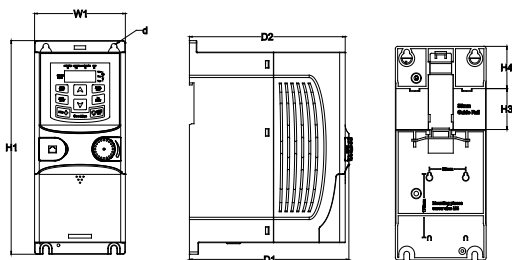
Abbildung B-5 Schienenmontage von Frequenzumrichtern der Kategorien 1PH 220 V/3PH 380 V ( \leq 2,2 kW) und 3PH 220 V ( \leq 0,75 kW) (Maßeinheit: mm)
