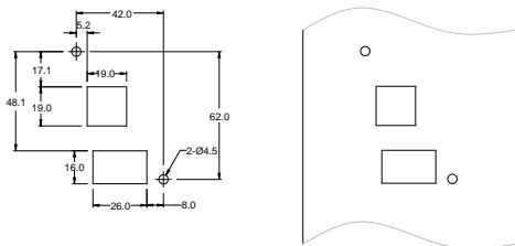
Abbildung B-2 Bohrschablone für Bedienfeld ohne Konsole.
