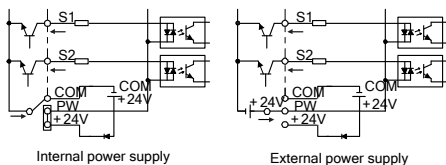
Abbildung 3-14 NPN-Betriebsarten
