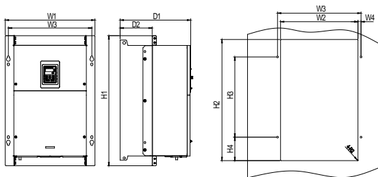
Abbildung B-10 Flanschmontage von Frequenzumrichtern der Kategorie 3PH 400 V 90–110 kW Abmessungen in mm
