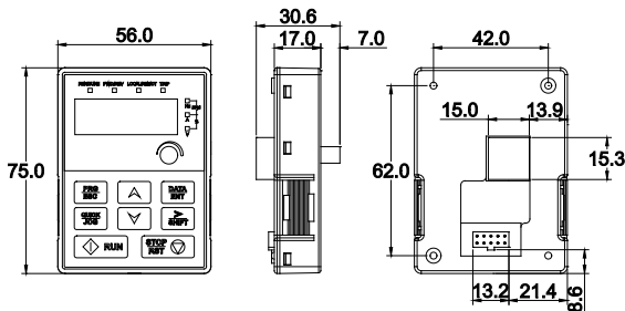
Abbildung B-1 Abmessungen des Bedienfelds
